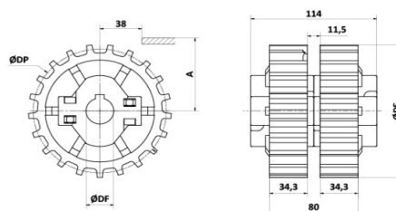
Piñón Asimétrico Serie 821 - Con chavetero - UNI 6604-69 / ISO 773 - DIN 6885
