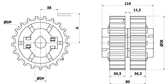
Piñón Asimétrico Serie 821 - Con chavetero - UNI 6604-69 / ISO 773 - DIN 6885
