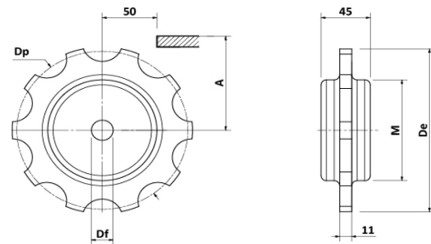
Piñón Serie 1700 - Sin chavetero
