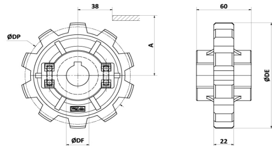
Piñón Serie 882 - Con chavetero - UNI 6604-69 / ISO 773 - DIN 6885
