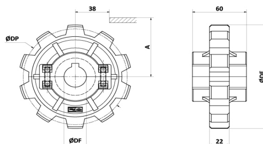
Piñón Serie 882 - Con chavetero - UNI 6604-69 / ISO 773 - DIN 6885
