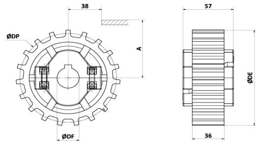
Piñón Serie 881 - Con chavetero - UNI 6604-69 / ISO 773 - DIN 6885
