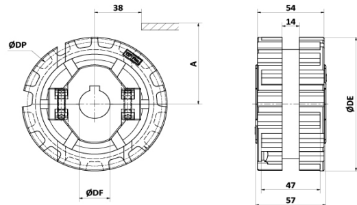
Piñón Serie 820 / 831 - Con chavetero - UNI 6604-69 / ISO 773 - DIN 6885
