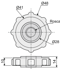
Perilla Ajuste Rosca 9/16" - 1/2" - M14 Knob 9/16" - 1/2" - M14
