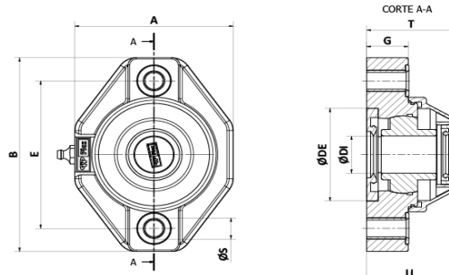
Caja porta rodamiento - 2 agujeros - Negro (UCFL) - Rodamiento (UC) / (S-UC) Inoxidable.
