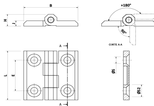
Bisagra Aluminio - Negro
