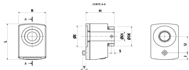
Posicionador Inclinado - superior / inferior - Naranja
