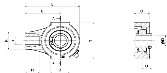
Caja porta rodamiento - Tensor - Fundición - Rodamiento acero al carbono (UCT)
