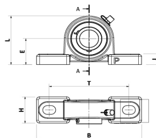
Caja porta rodamiento - Omega - Fundición - Rodamiento acero al carbono (UCP)
