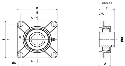
Caja porta rodamiento - 4 agujeros - Inoxidable - Rodamiento Inoxidable (SUCF)
