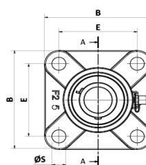
Caja porta rodamiento - 4 agujeros - Fundición - Rodamiento acero al carbono (UCF)
