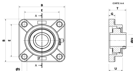
Caja porta rodamiento - 4 agujeros - Blanco - Rodamiento Inoxidable (UCF)
