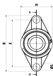
Caja porta rodamiento - 2 agujeros - Inoxidable - Rodamiento Inoxidable (SUCFL)
