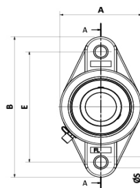
Caja porta rodamiento - 2 agujeros - Blanco - Rodamiento Inoxidable (UCFL)
